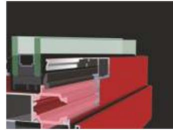
Thermal break strip
